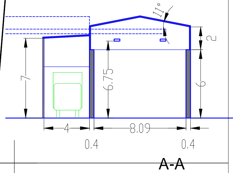
SCHEMATY PRZEKROJÓW 1:200
